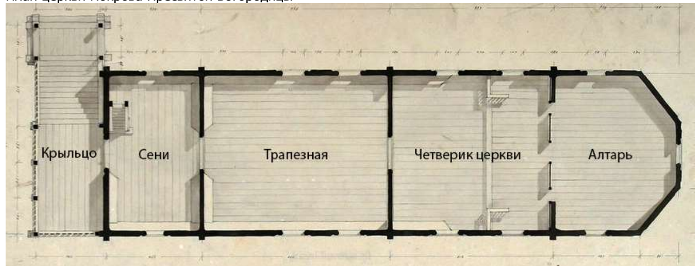
План церкви Покрова Пресвятой Богородицы
