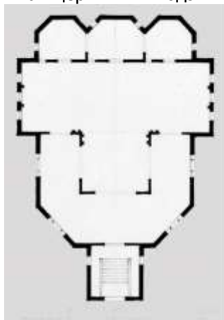
План церкви А.Б.Бодэ
