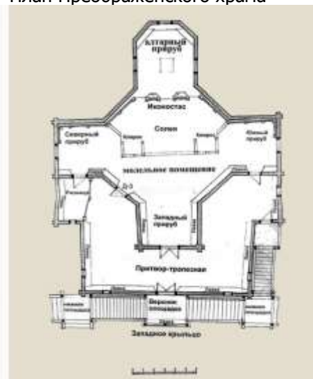
План Преображенского храма
